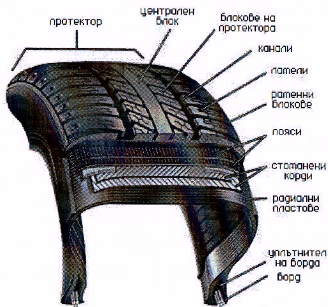
Структура на радиална автомобилна гума
